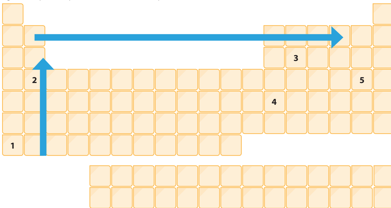
Figura 2: Propiedades periódicas de los elementos químicos.
